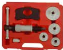
7pc Brake caliper piston tools set ชุดเครื่องมือกดลูกสูบดิสเบรคแบบเกลียว 7 ชิ้น
